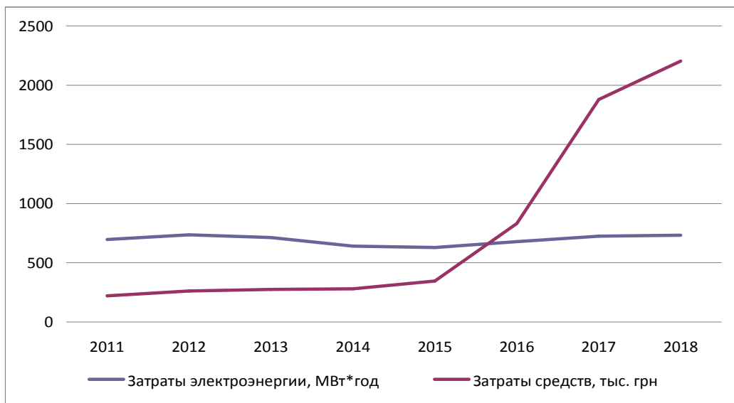
Графік 1. Вартість електроенергії та засоби зовнішнього освітлення міста (2011-2018 рр)
